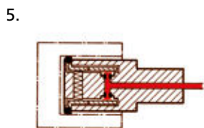
5. Měření průměrů slepých otvorů s hlavicí s kuličkovými kontakty
